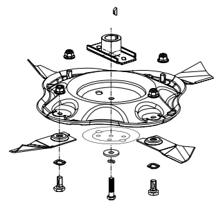
Quadcut®-kniv
