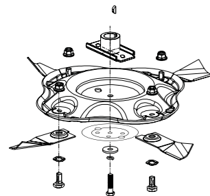
Lâmina Quadcut®
